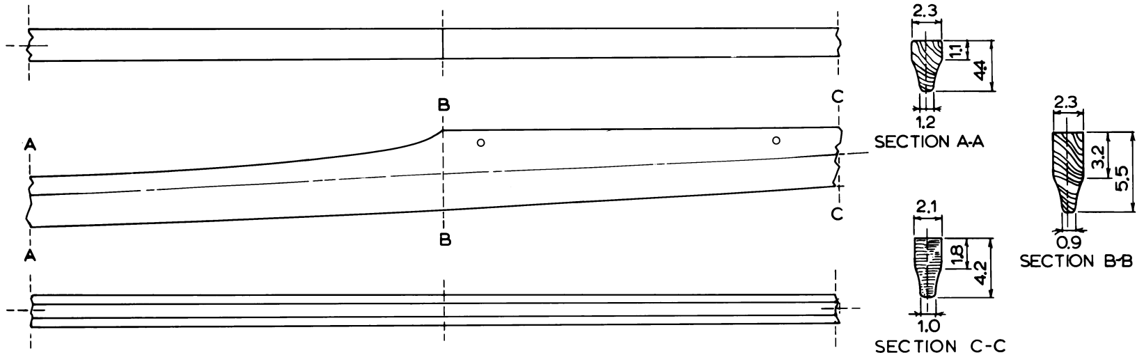
STERN KEELSON PIECE
