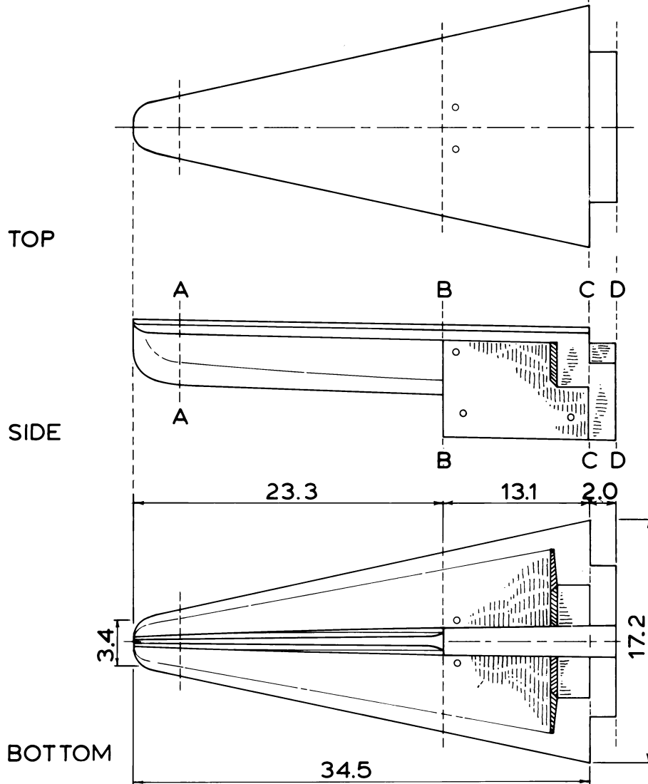
UPPER STEM PIECE
